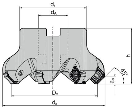
Fresa a manicotto 45° / SN.. 12 Fresa de planeado 45° / SN.. 12
